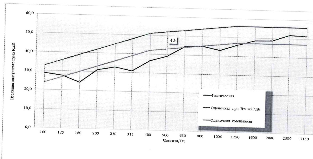
Рис. 3 Спектр изоляции фрагмента перегородки «базовая конструкция + бескаркасная конструкция для дополнительной звукоизоляции стен (модуль №2)»
