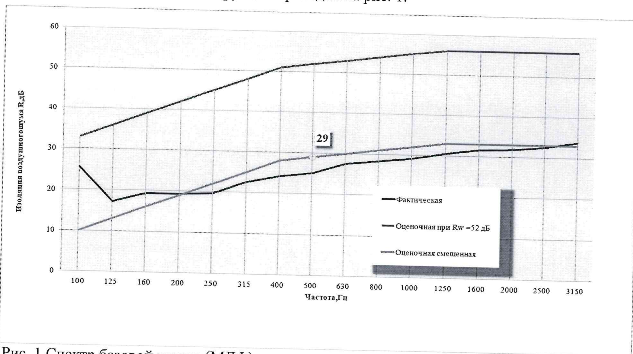
Рис. 1 Спектр базовой плиты (МДФ)
