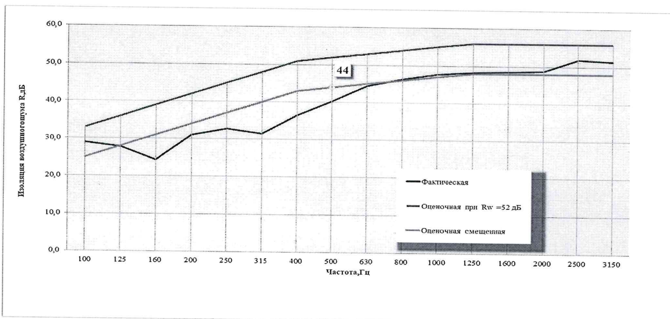
Рис. 3 Спектр изоляции фрагмента перегородки «базовая конструкция + бескаркасная конструкция для дополнительной звукоизоляции стен (модуль №3)»
