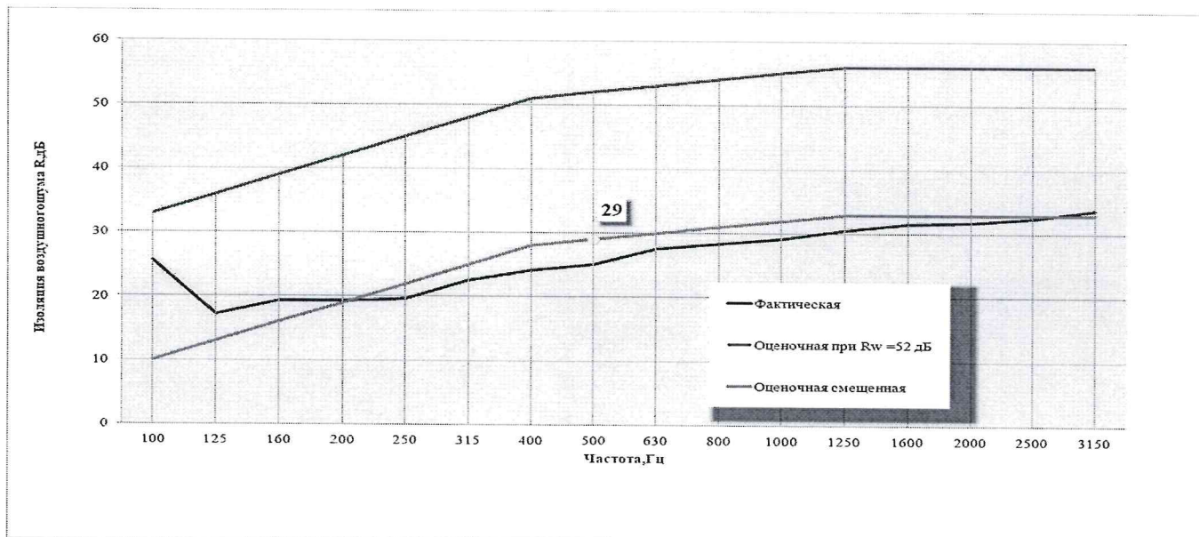
Рис. 1 Спектр базовой плиты (МДФ)
