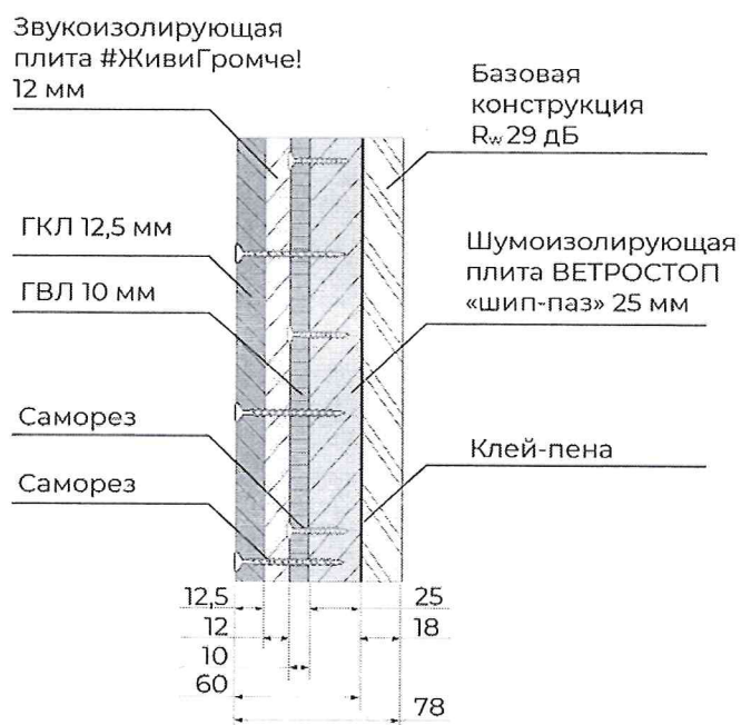
Рис. 2 Эскиз конструкции для дополнительной звукоизоляции (модуль №3)
